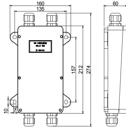
14: SG-1A 继电器盒 relay box
